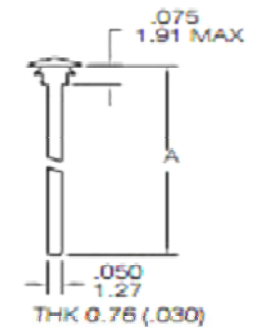
PCB Terminal Option (C) + (D)
