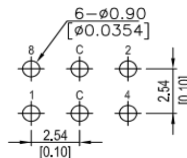
P.C.B. Layout (mm)
