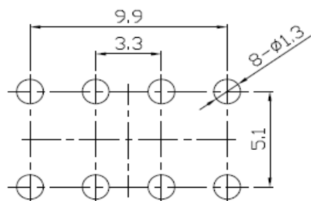
P.C.B Layout (mm)
