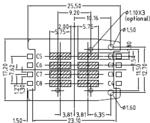
P.C.B. Layout 8PIN
