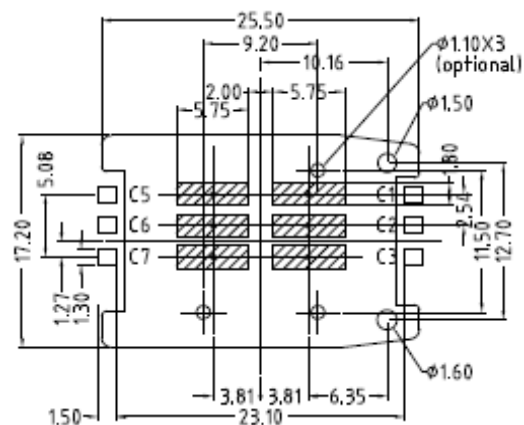
P.C.B. Layout 6PIN
