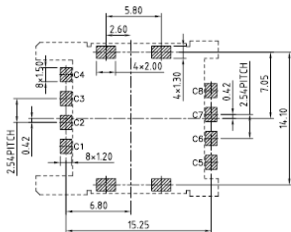
P.C.B. Layout 8PIN
