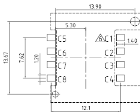
P.C.B. Layout 8Pin
