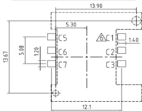
P.C.B. Layout 6Pin
