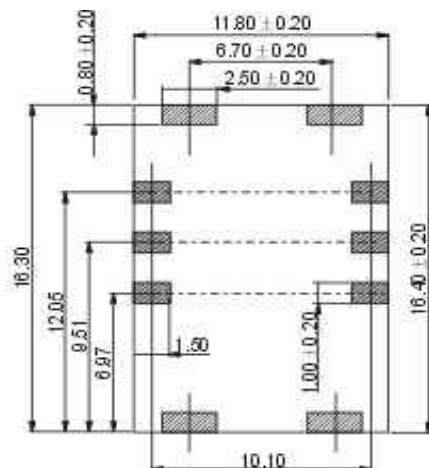
P.C.B. Layout 6Pin
