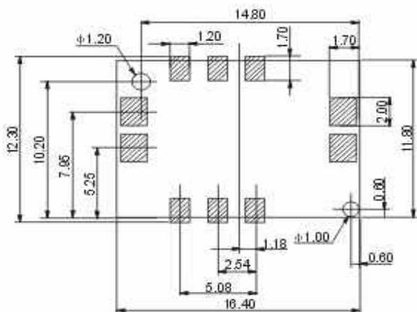
P.C.B. Layout 6Pin
