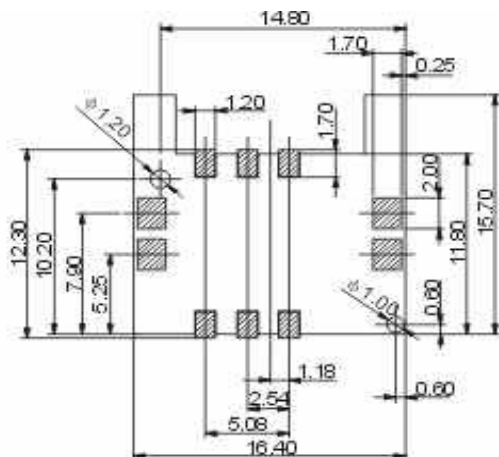
P.C.B. Layout 6Pin
