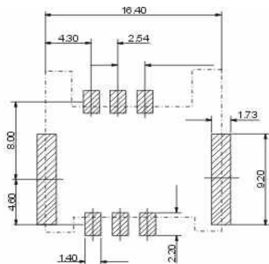
P.C.B. Layout 6Pin
