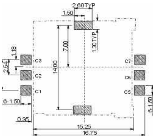
P.C.B. Layout 6Pin
