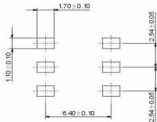
P.C.B. Layout 6Pin
