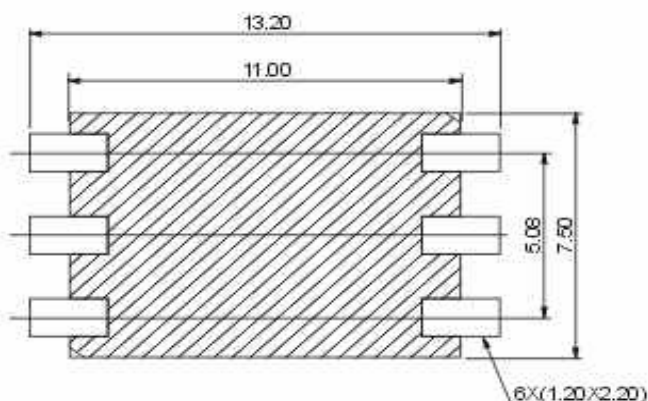
P.C.B. Layout 6Pin
