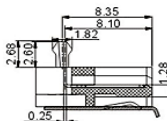
SECT A-A
