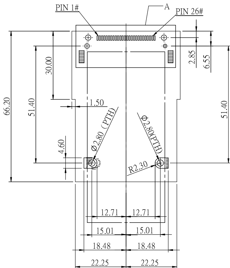
細部放大圖 A 比例 2 : 1
