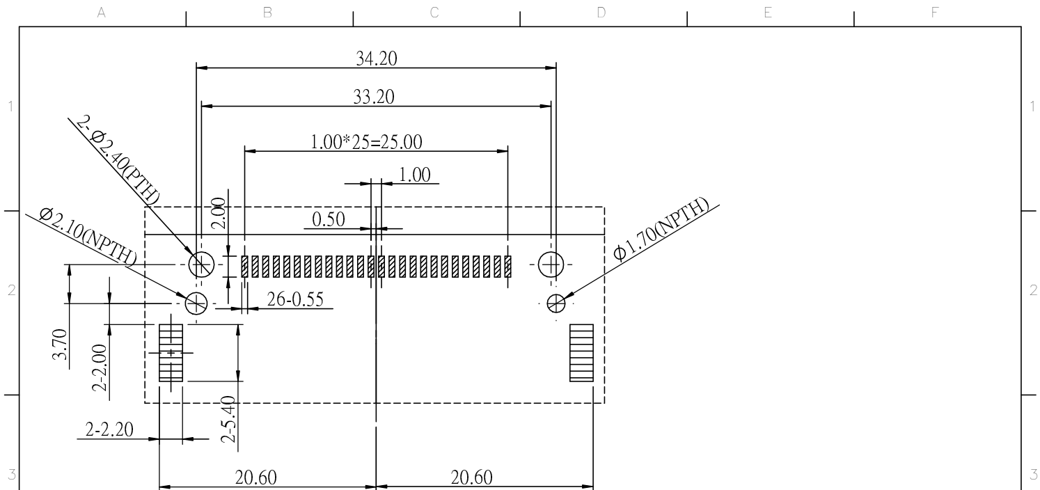
細部放大圖 A 比例 2 : 1
