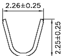
SEC:A-A
