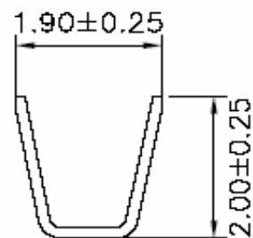
SEC:A-A
