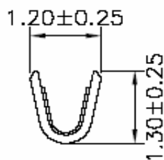
SEC:B-B
