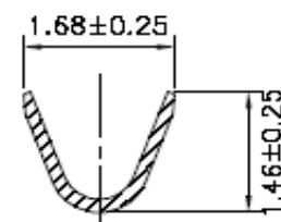
SEC:A-A
