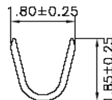
SEC:A-A
