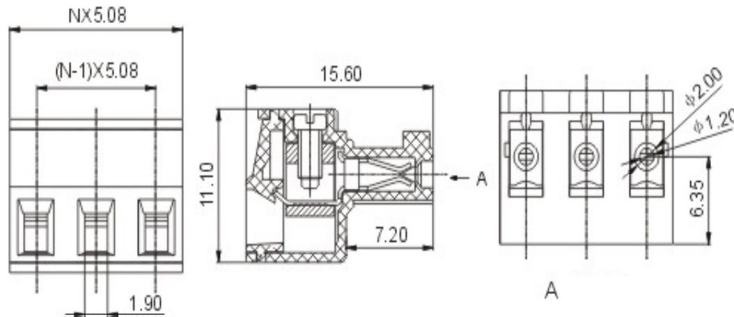
P.C.B. Layout
