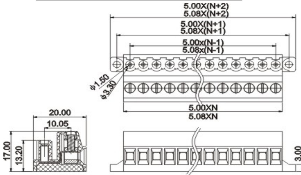
P.C.B. Layout
