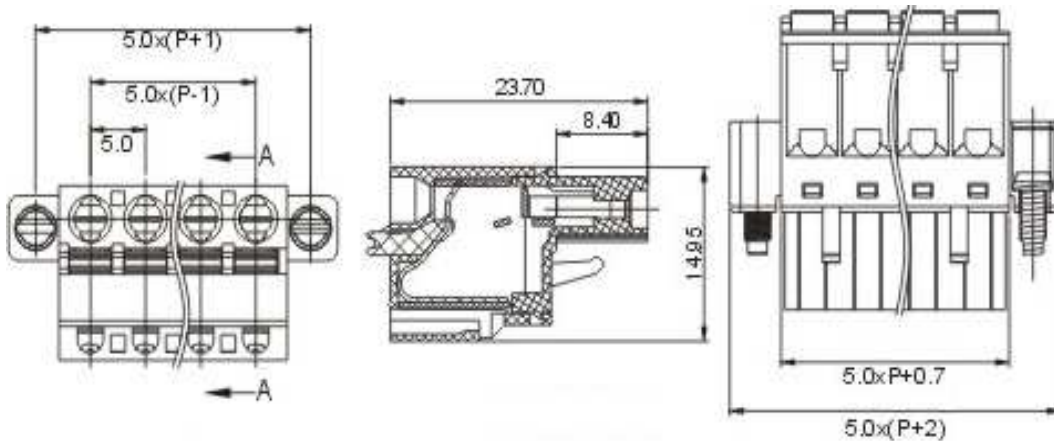
P.C.B. Layout
