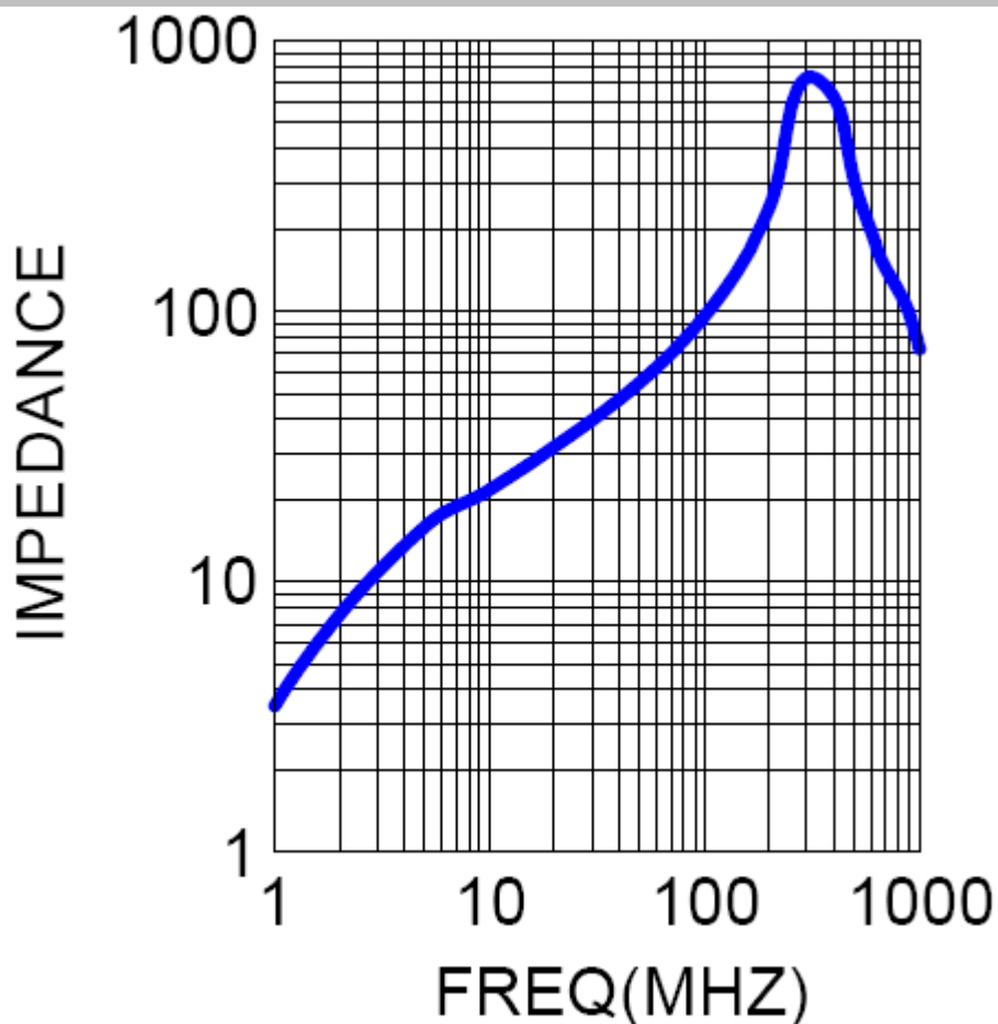
Material A5
