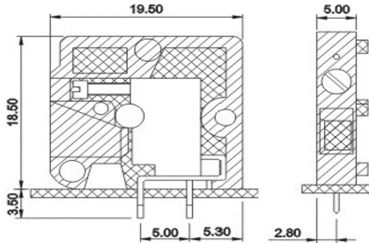
P.C.B. Layout
