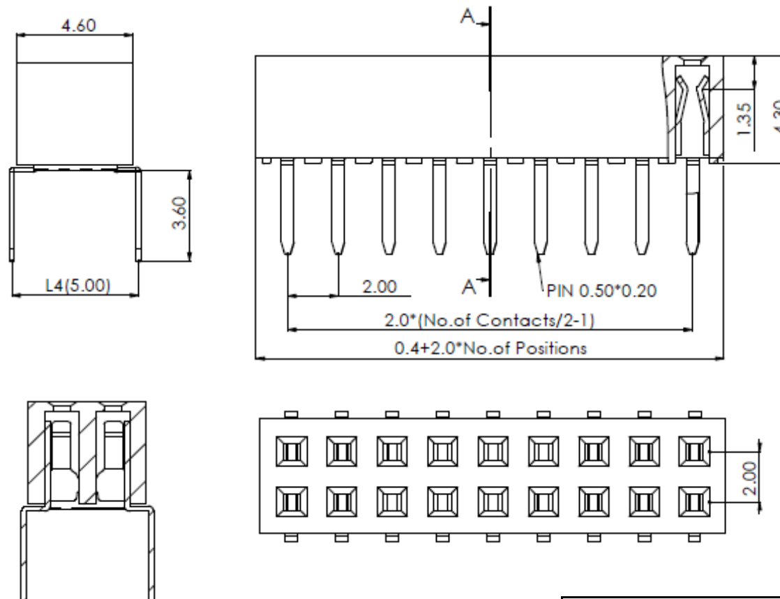
SECTION A-A
