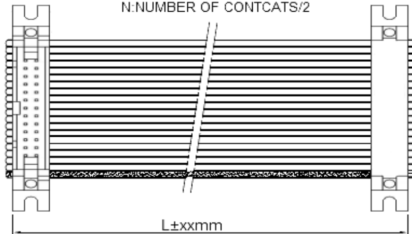
Typ A5
