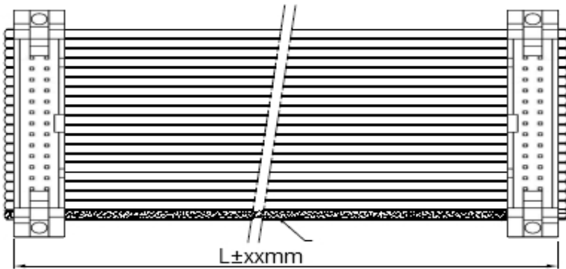
Typ A1
