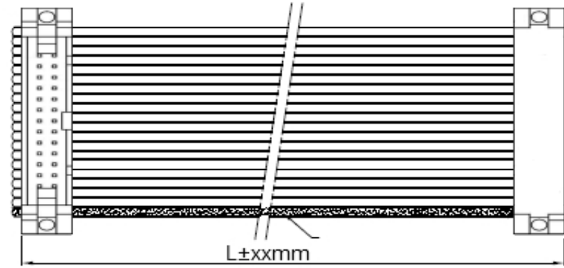
Typ A4
