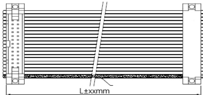
Typ A5
