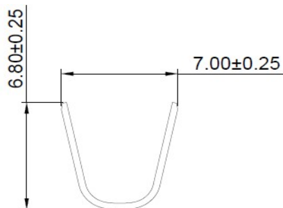
SEC:A-A
