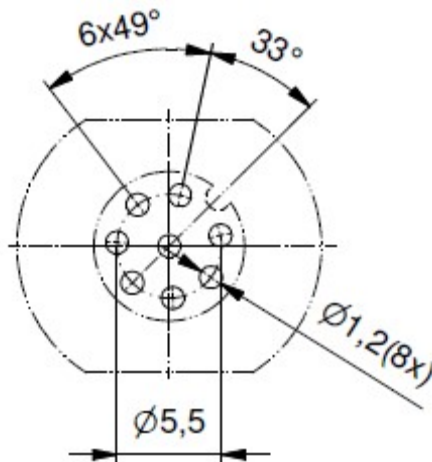
PCB-Layout 8Pos.
