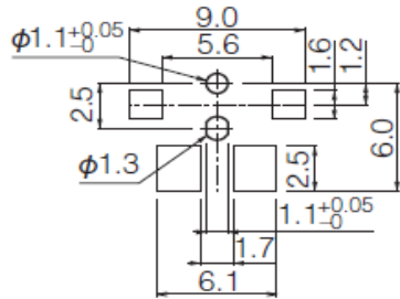
P.C.B Layout (mm)
