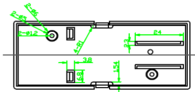
下壳俯视图
