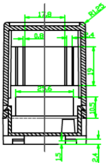
截面 B-B
