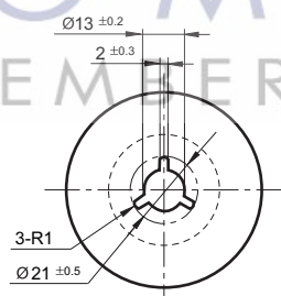
Reel Dimensions
